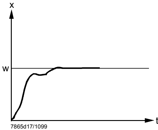
Иллюстрация 33: Pb слишком мал
