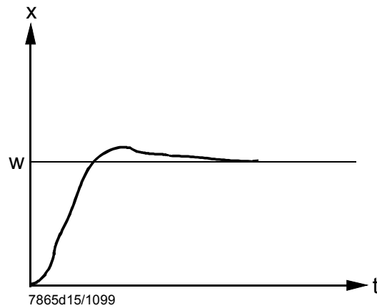
Иллюстрация 34: Pb слишком велик
