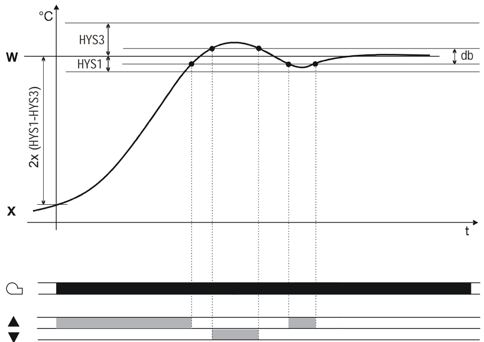
Иллюстрация 18: Программируемый цикл, холодный пуск оборудования
