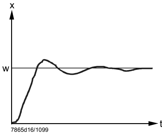
Иллюстрация 35: rt, dt слишком малы
