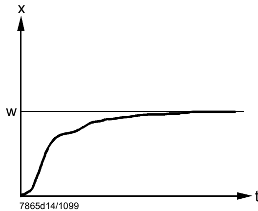
Иллюстрация 36: rt, dt слишком велики
