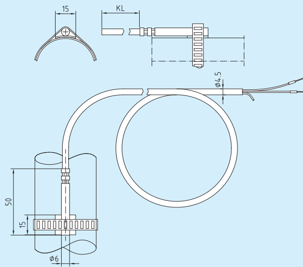
Габаритный чертеж
